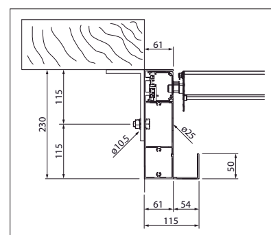
TR4520 Intersección del perfil de la viga( Anclado arriba )
