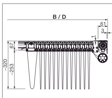
TR4110 Vista lateral en detalle
