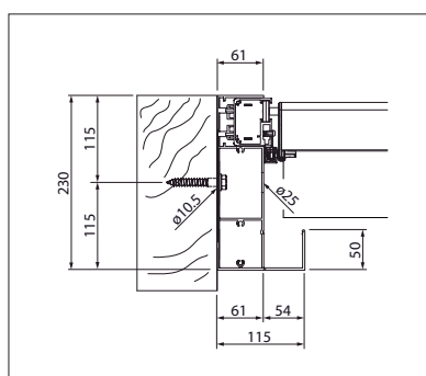
TR4120 Intersección del perfil de la viga(montaje entre paredes)
